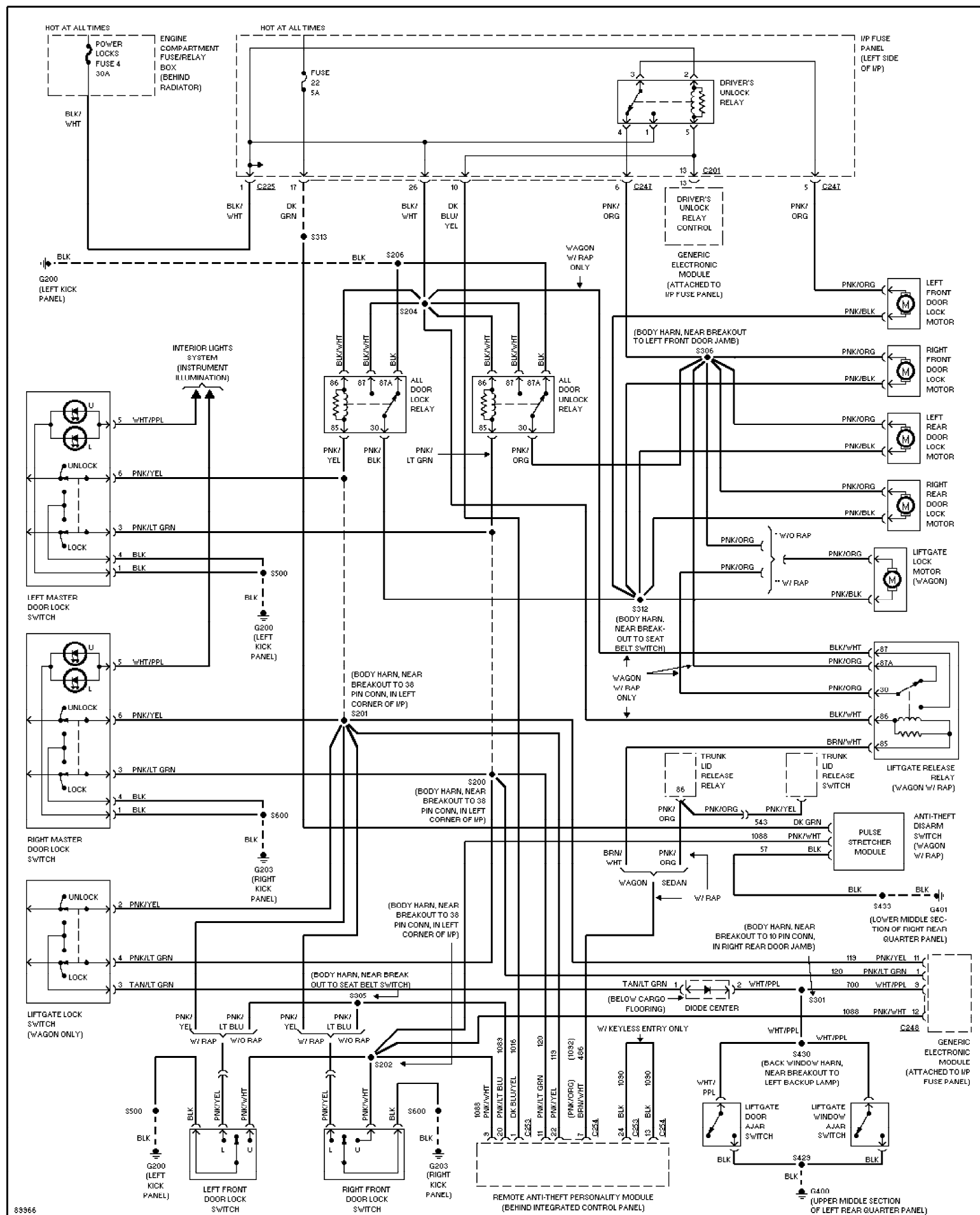
Fig. 54: Power Door Lock Circuit 1997 Ford Taurus LX
