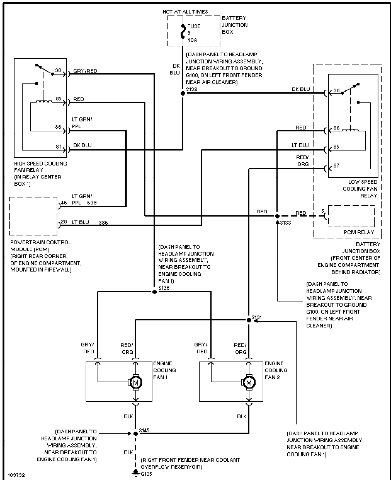
Fig. 9: Cooling Fan Circuit 1999 Ford Taurus LX
