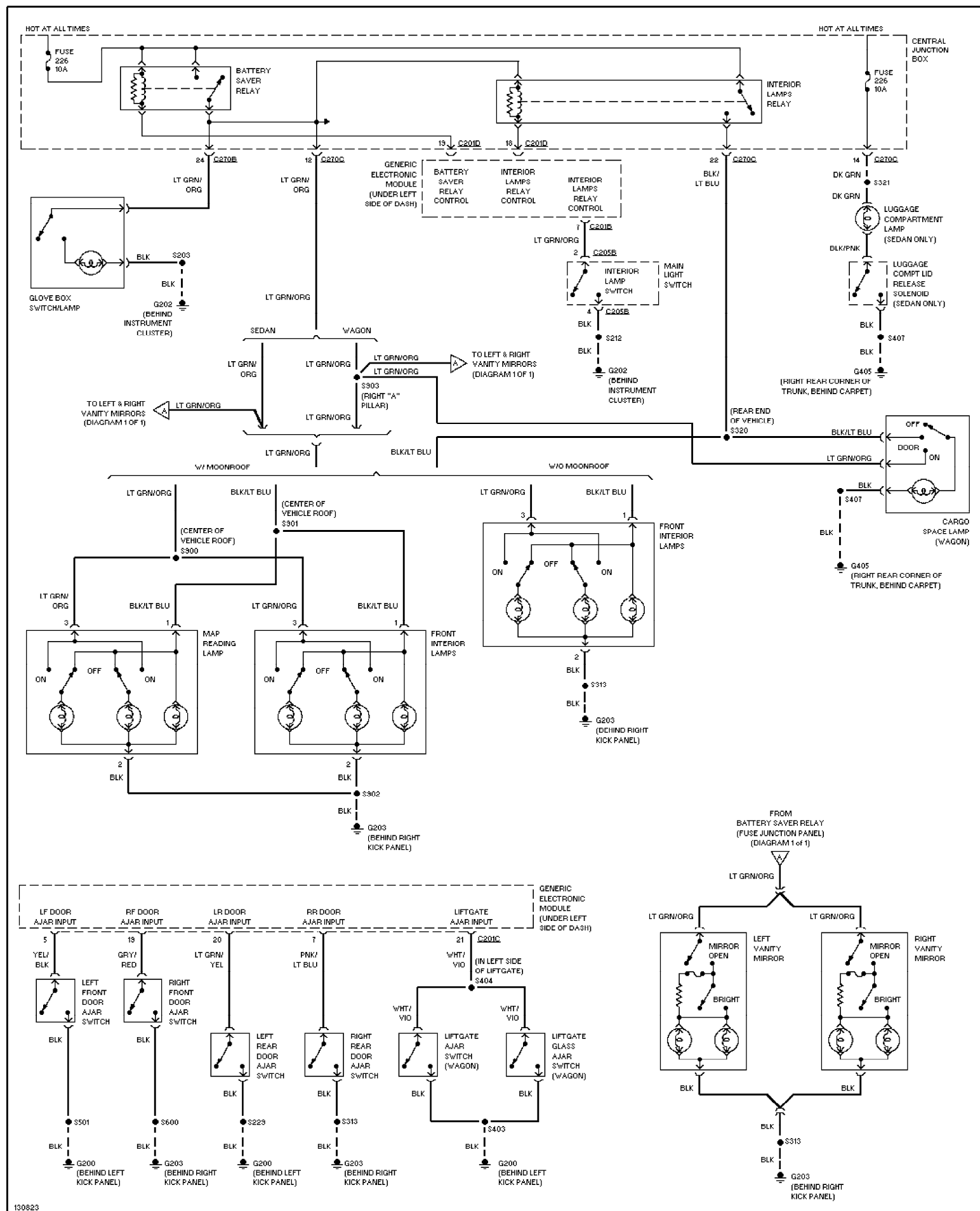
Fig. 37: Courtesy Lamps Circuit 2000 Ford Taurus SES
