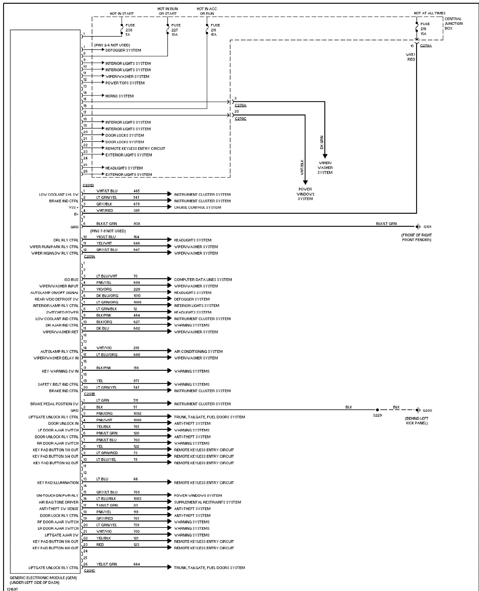
Fig. 8: Body Computer Circuits 2000 Ford Taurus SES
