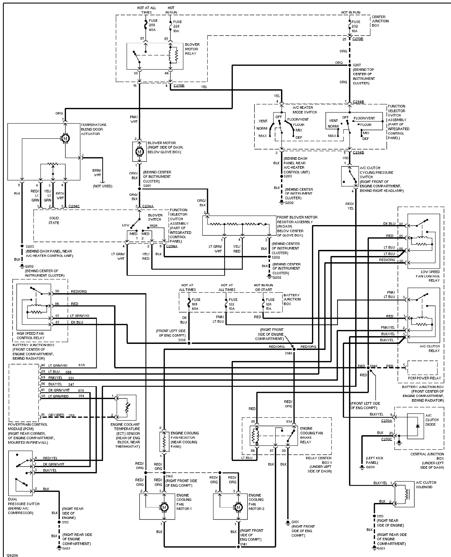
Fig. 3: Manual A/C Circuit 2000 Ford Taurus SES
