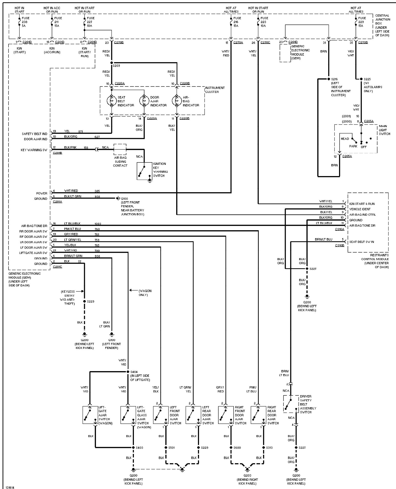
Fig. 59: Warning System Circuits 2000 Ford Taurus SES
