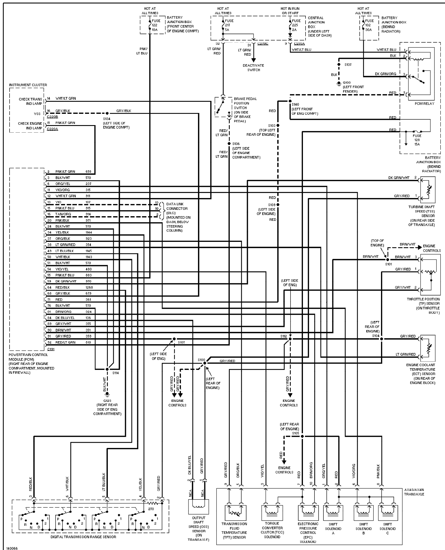
Fig. 56: 3.0L 24-Valve, A/T Circuit 2000 Ford Taurus SES
