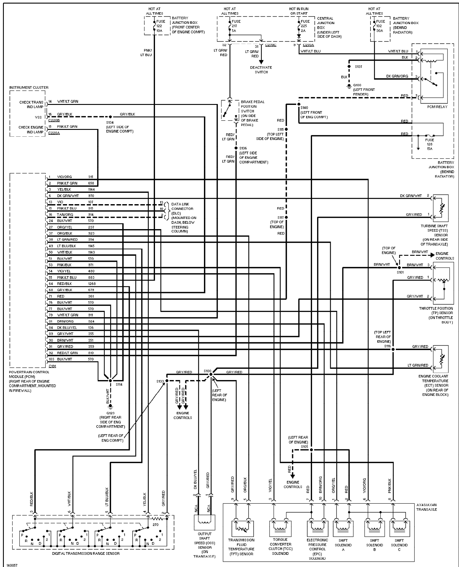
Fig. 57: 3.0L Flex Fuel, A/T Circuit 2000 Ford Taurus SES
