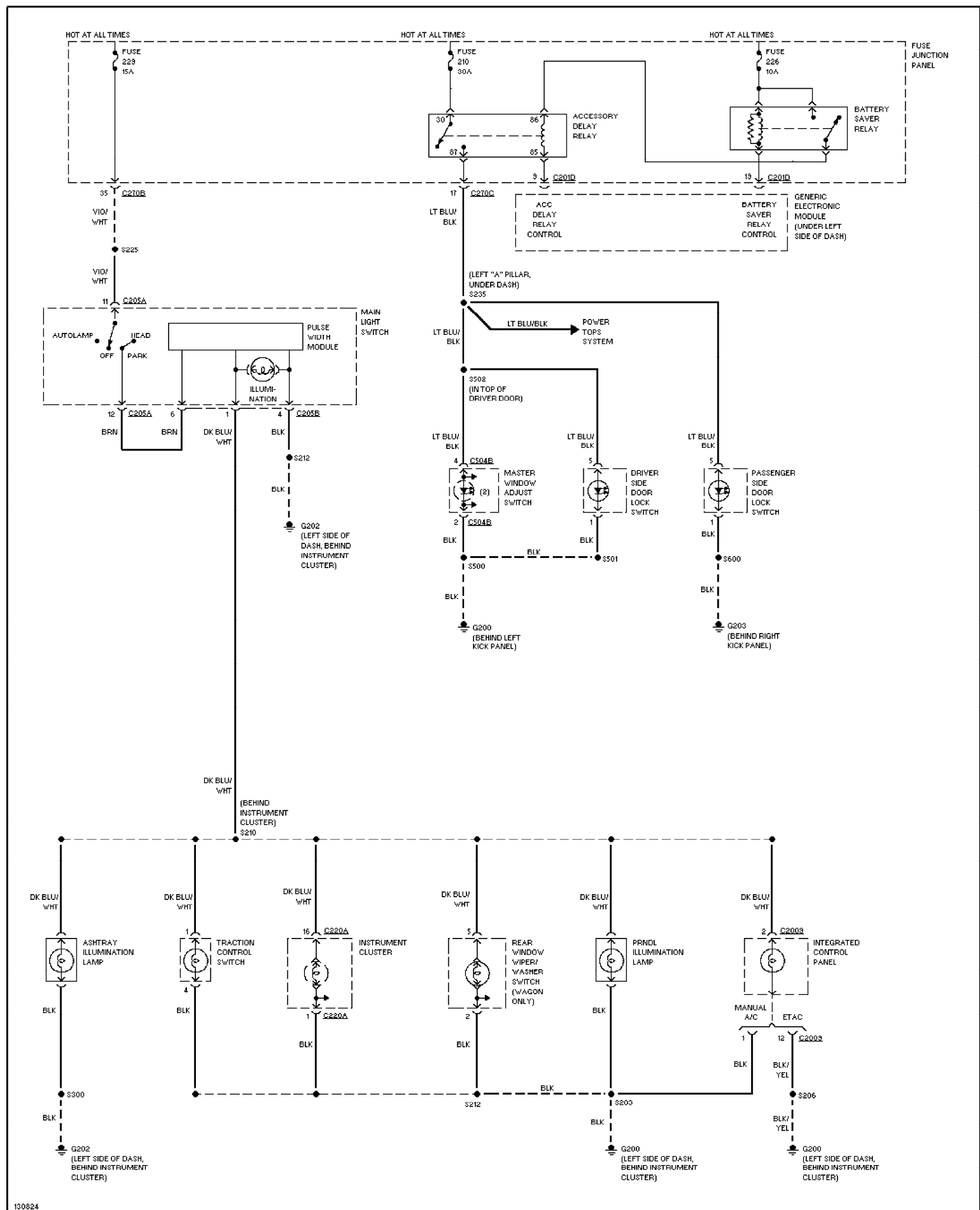
Fig. 38: Instrument Illumination Circuit 2000 Ford Taurus SES
