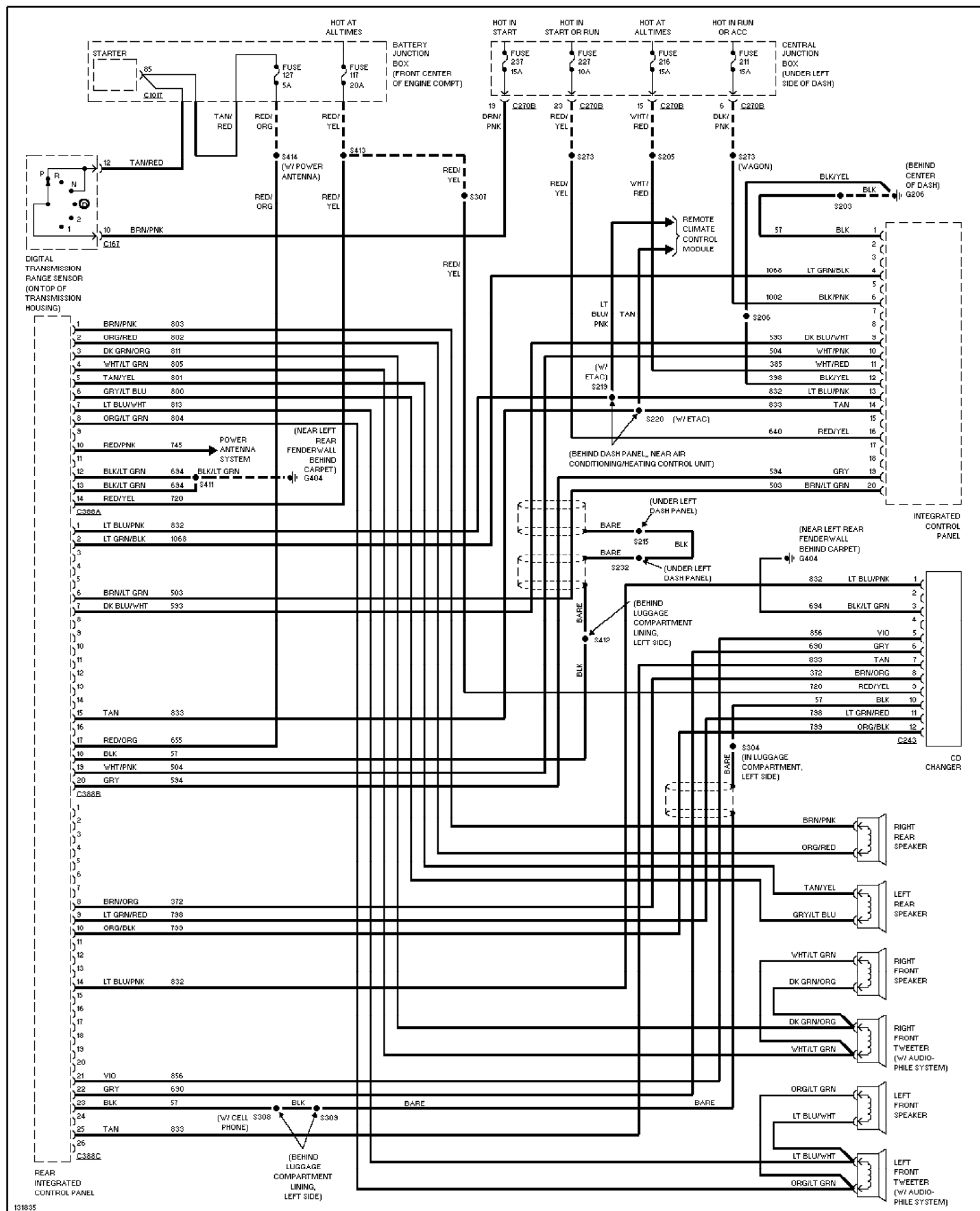
Fig. 50: Radio Circuits 2001 Ford Taurus SEL
